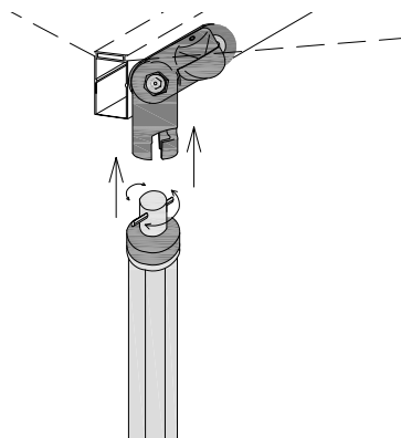
-Detalle instalación a parasol
