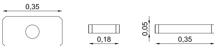
-Detalle regleta (comprobar que cabe en la barra del toldo)
