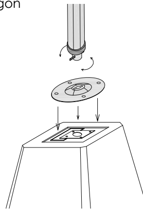
-Detalle instalación pata a peso de hormigón
