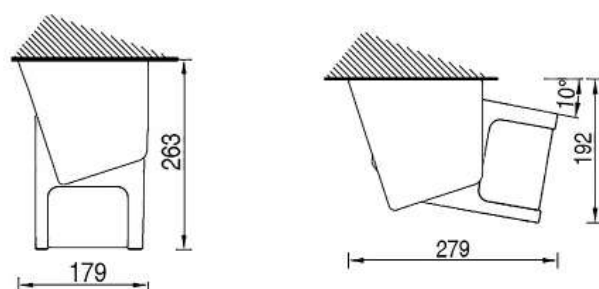
Dimensiones soporte a techo
