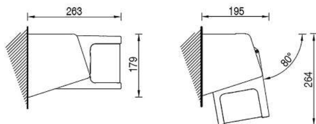
Dimensiones soporte a pared
