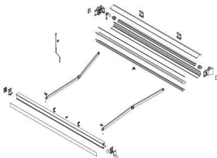
Qubica Light despiece
