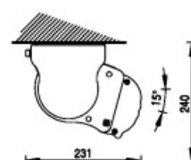
Montaje a techo 15°
