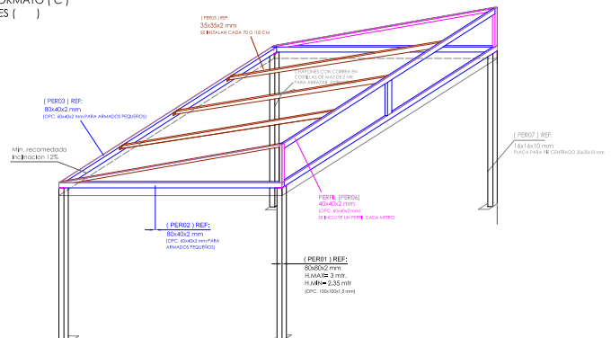
ESQUEMA ORIENTATIVO ARMADO TIPO / FORMATO ( C ) Nº DE PIES: ( )
