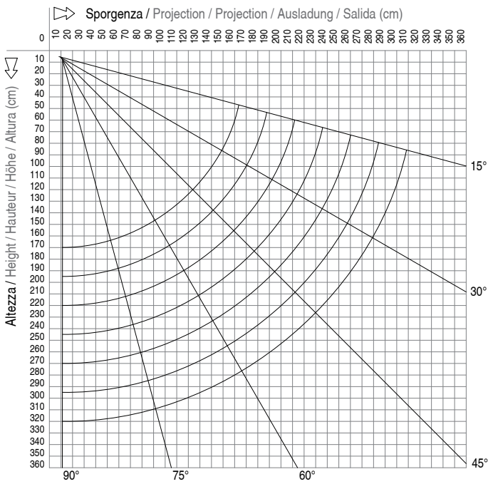
Diagrama de proyección - Montaje a techo Covering diagram - Ceiling installation
